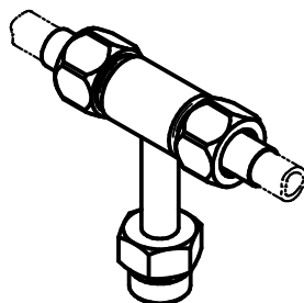
Fig.121 Zwischenhalter für Anzeiger Fig.121 Holder for fluid-level indicator G3/4" -20°C / +200°C
