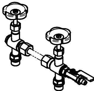
Fig.127 Ventilflüssigkeitsstand-Anzeiger Fig.127 Valve fluid-level indicator G1/2" -20°C / +200°C
