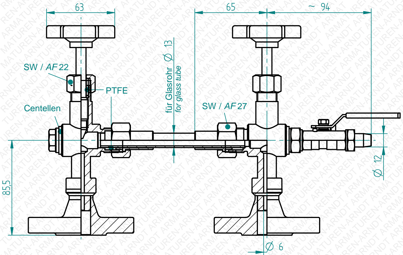
Flanschabmessungen flange dimensions
